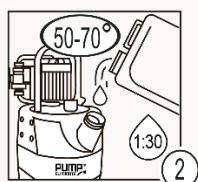
Шаг 2. Подготовить промывочный раствор
