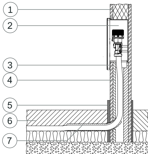
Рис. 5: Монтаж в сечении
